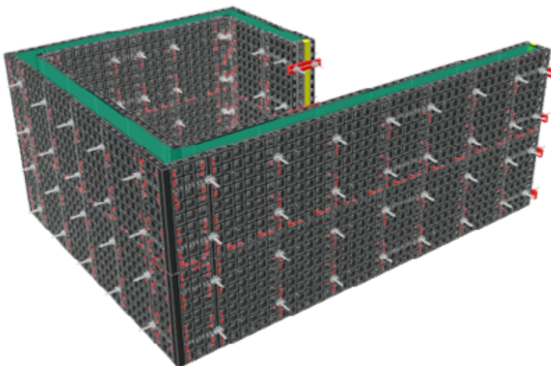
Beispielhafte Grundrissplanung aus dem QuickSolve Planer (b = 25 cm, h = 270 cm)
